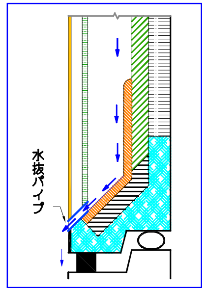
施工断面例
